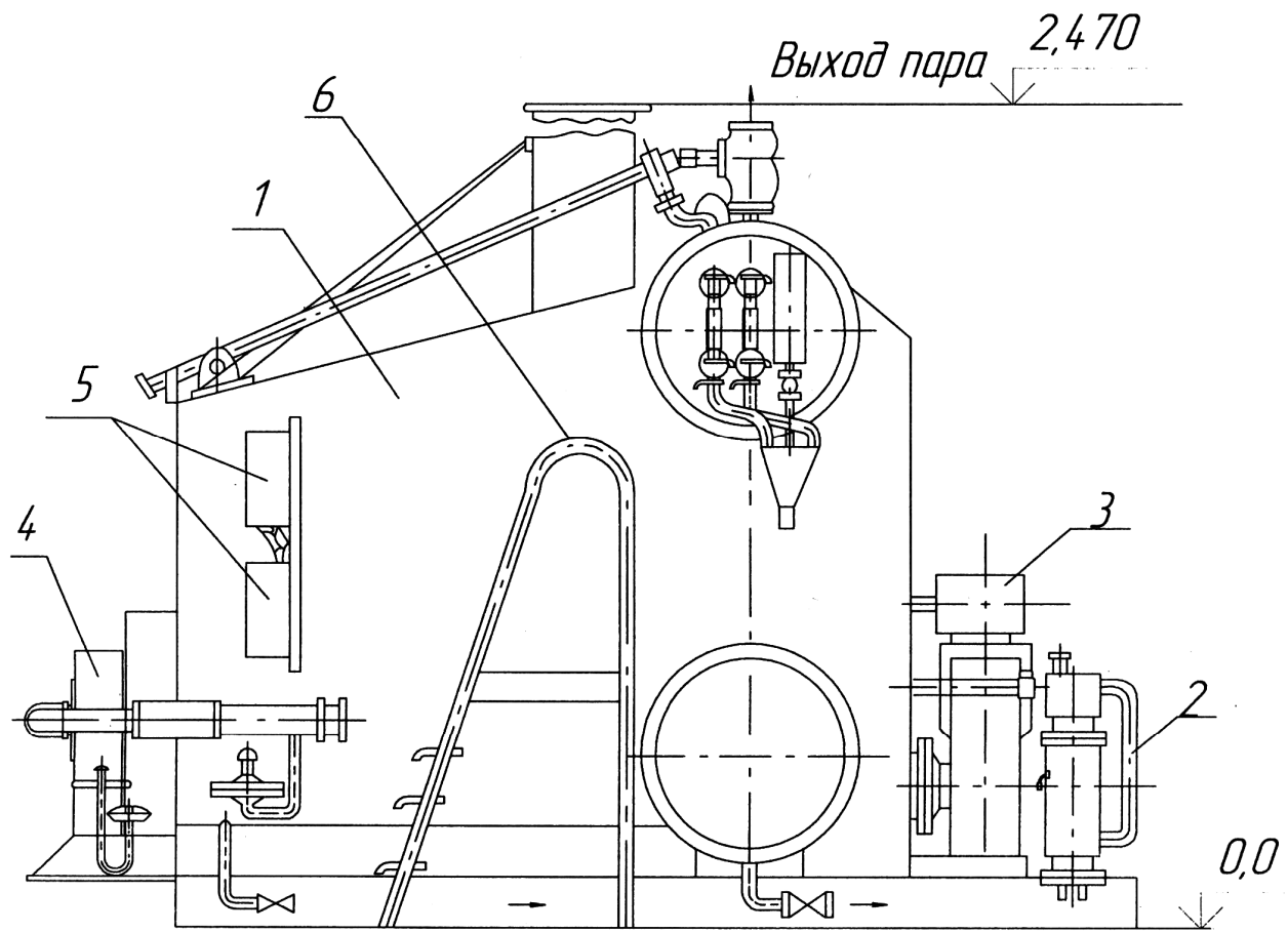
Рис.1, Котел паровой E-1,0-0,9Г-3(Э)
