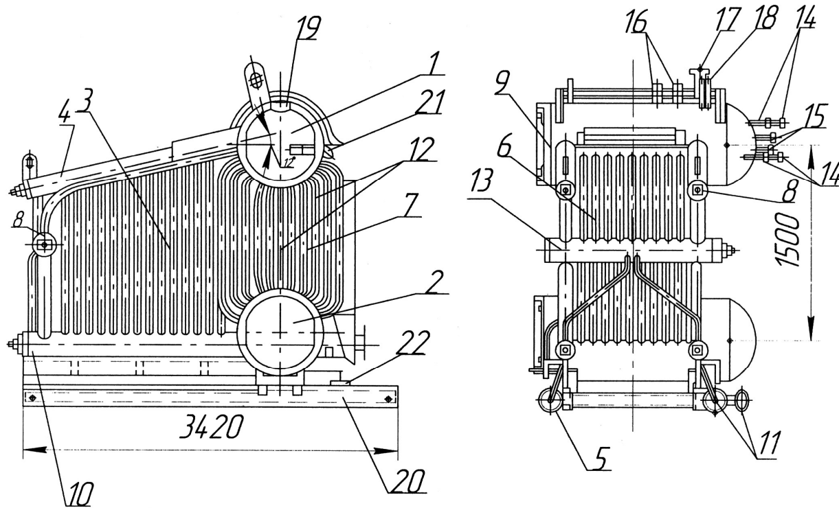
Рис. 2, Трубная система
