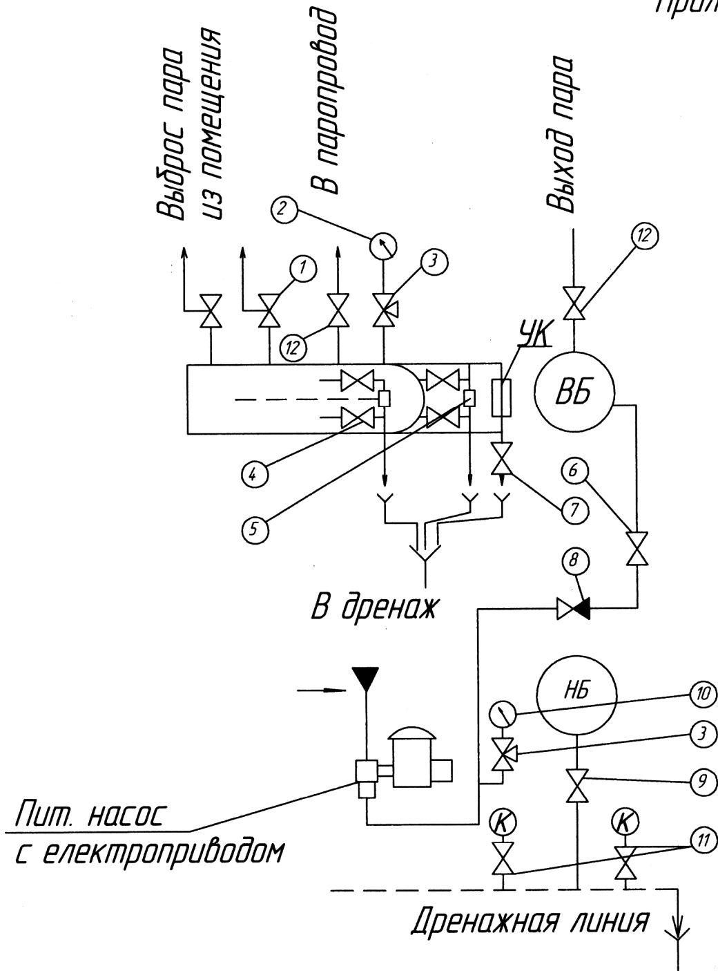
Рис. 4. Схема трубопроводов
