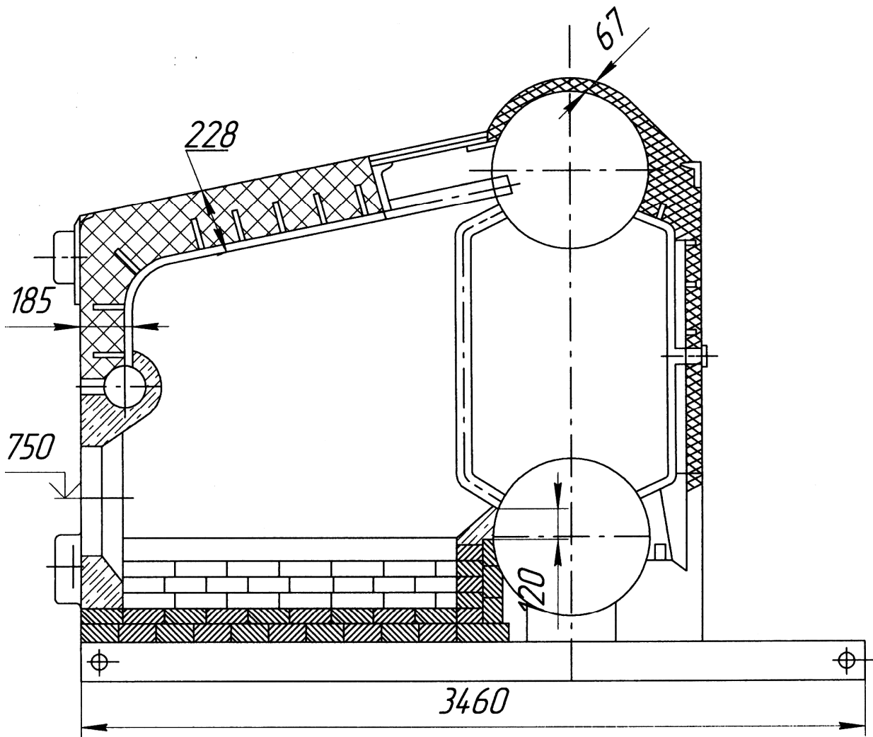
Рис. 3, Теплоизоляция
